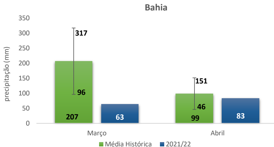
Figura 11 Média histórica das fazendas da Bahia versus a precipitação medida nas fazendas da Bahia (SLC)
