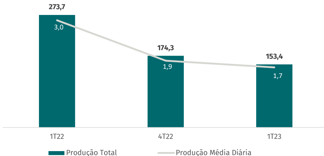
Gráfico 16 – Produção total de gás, em MMm³, e produção média diária, em MMm³/dia, do Campo de Manati
