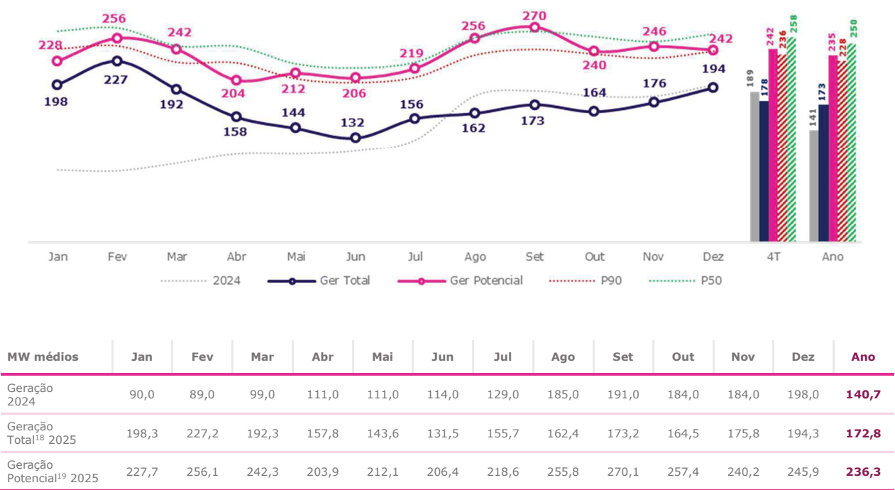
Ativos Solares – Geração de Energia e Valores Certificados para o P50 e P90 (MW médios)
