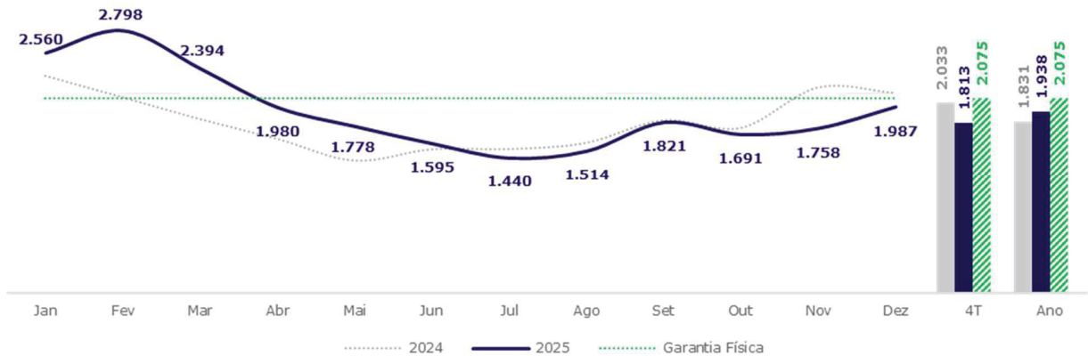
Geração de Energia e Valores de Garantia Física (MW médios) 8
