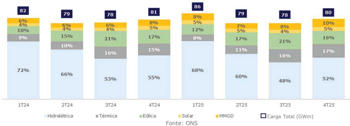
Balanco Energético (SIN) – Contribuição por Fonte para Atendimento à Carga (GW médios)
