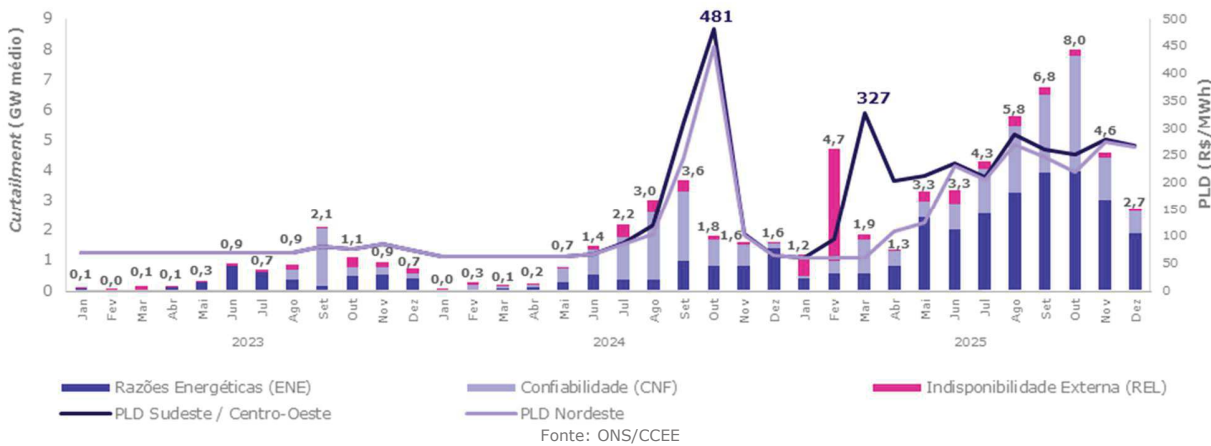
Curtailment Eólico e Solar (GW médio) e PLD (R$/MWh)
